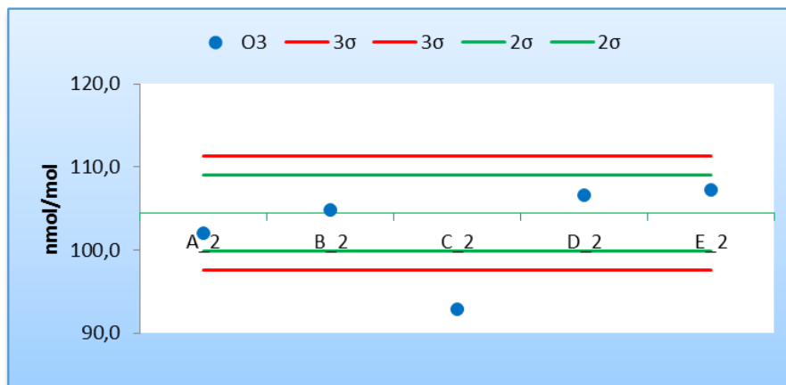
Figura 4 - Resultados y cumplimiento de los criterios de aceptación de sesgo de los laboratorios participantes para la concentración c3 de O 3 (104,43 nmol/mol)
