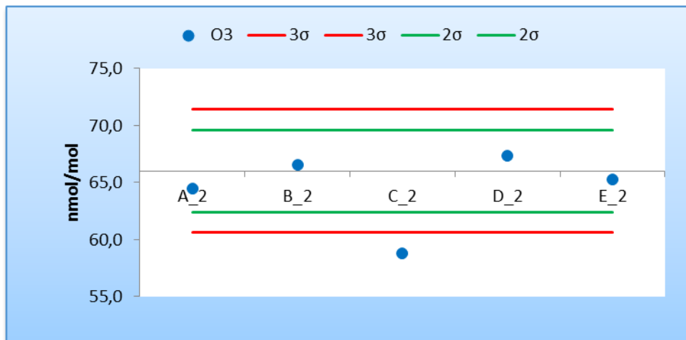
Figura 6 - Resultados y cumplimiento de los criterios de aceptación de sesgo de los laboratorios participantes para la concentración c5 de O 3 (66,01 nmol/mol)
