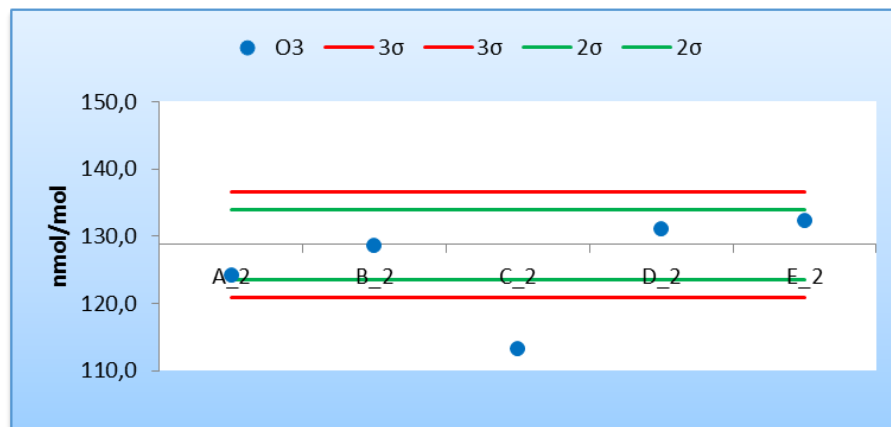
Figura 2 - Resultados y cumplimiento de los criterios de aceptación de sesgo de los laboratorios participantes para la concentración c1 de O 3 (128,72 nmol/mol)
