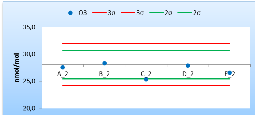
Figura 3 - Resultados y cumplimiento de los criterios de aceptación de sesgo de los laboratorios participantes para la concentración c2 de O 3 (28,05 nmol/mol)
