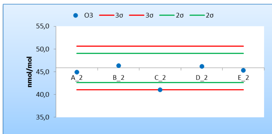
Figura 5 - Resultados y cumplimiento de los criterios de aceptación de sesgo de los laboratorios participantes para la concentración c4 de O 3 (45,85 nmol/mol)
