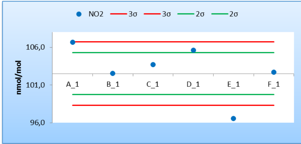
Figura 6 - Resultados y cumplimiento de los criterios de aceptación de sesgo de los laboratorios participantes para la concentración c1 de NO 2 (102,51 nmol/mol)
