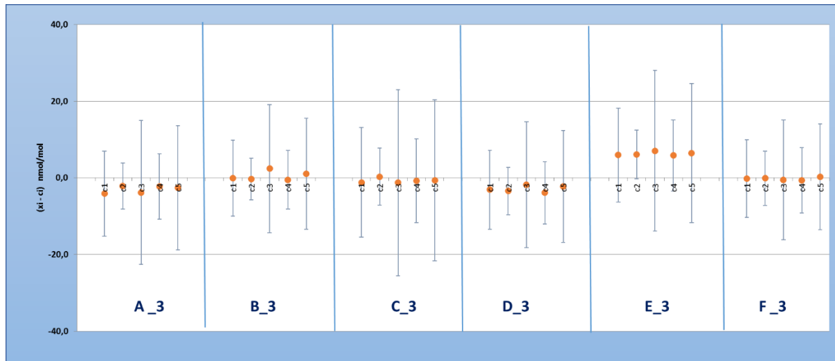
Figura 14.- Representación gráfica del sesgo de cada participante |x_i - c_i| con respecto al denominador de la ecuación del estadístico E_n para las concentraciones de \text{NO}_2
