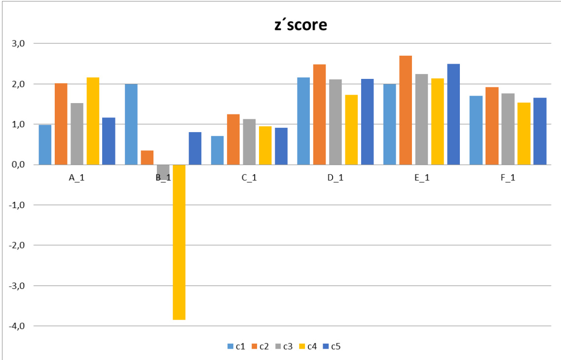
Figura 11 - Resultados de z'score para todos los participantes y todas las concentraciones de NO ensayadas
