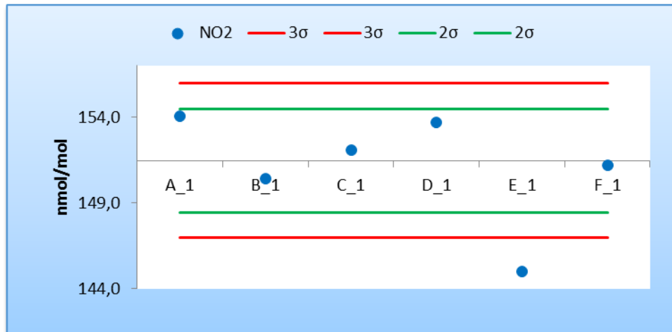
Figura 10 - Resultados y cumplimiento de los criterios de aceptación de sesgo de los laboratorios participantes para la concentración c5 de NO 2 (151,46 nmol/mol)
