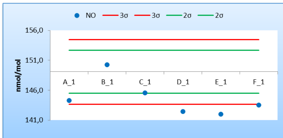
Figura 3 - Resultados y cumplimiento de los criterios de aceptación de sesgo de los laboratorios participantes para la concentración c3 de NO (149,08 nmol/mol)
