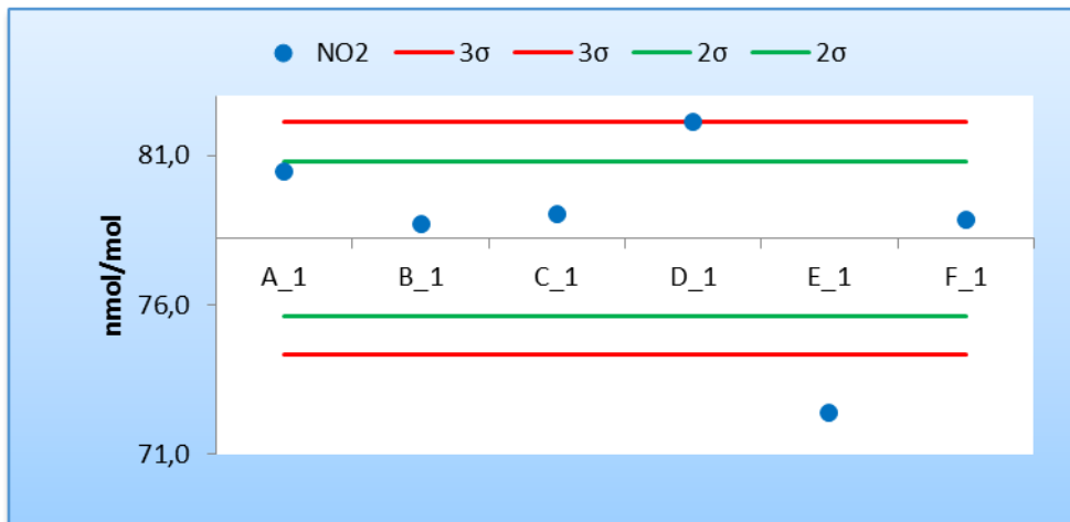
Figura 9 - Resultados y cumplimiento de los criterios de aceptación de sesgo de los laboratorios participantes para la concentración c4 de NO 2 (78,82 nmol/mol)
