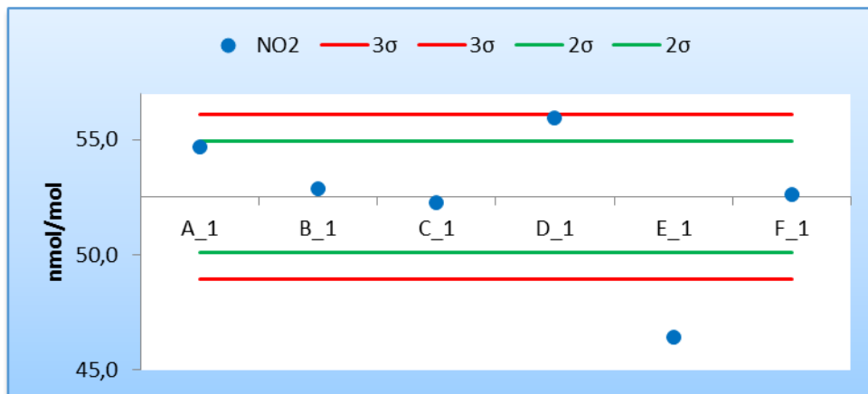
Figura 7 - Resultados y cumplimiento de los criterios de aceptación de sesgo de los laboratorios participantes para la concentración c2 de NO 2 (52,52 nmol/mol)
