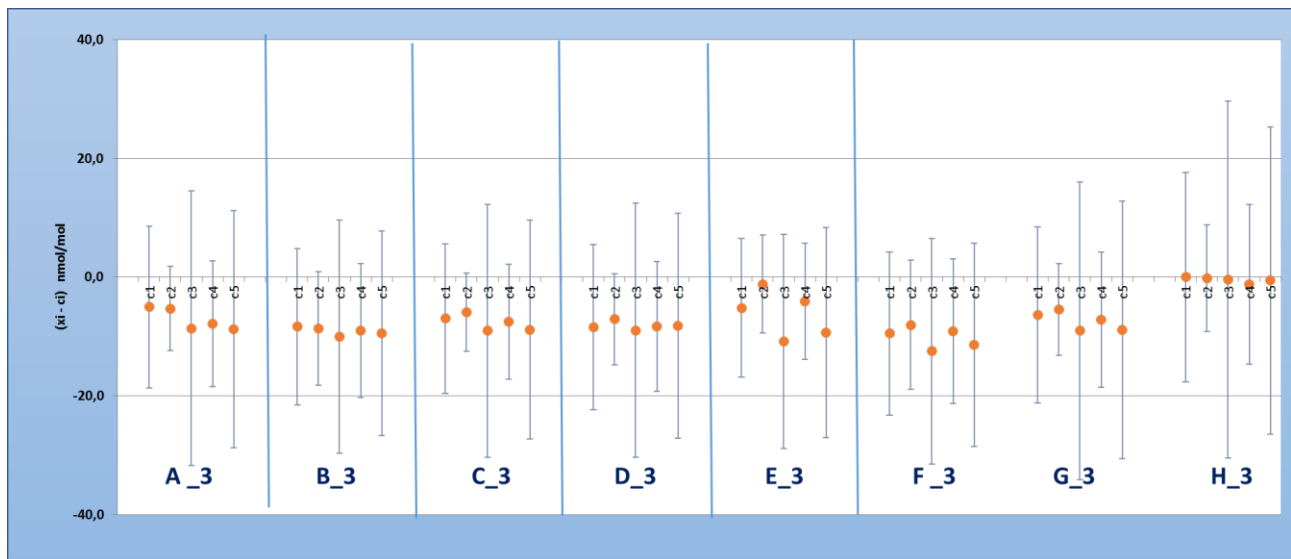
Figura 5.- Representación gráfica del sesgo de cada participante |x_i - c_i| con respecto al denominador de la ecuación del estadístico E_n para las concentraciones de \text{NO}_2
