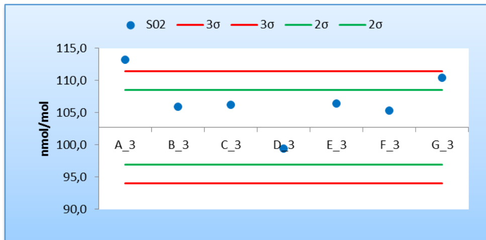
Figura 5 - Resultados y cumplimiento de los criterios de aceptación de sesgo de los laboratorios participantes para la concentración c4 de SO 2 (26,79 nmol/mol)
