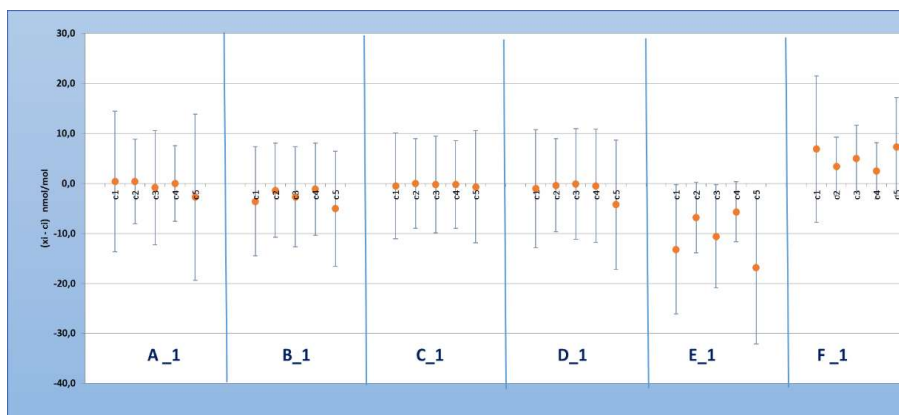
Figura 15.- Representación gráfica del sesgo de cada participante |x_i - c_i| con respecto al denominador de la ecuación del estadístico E_n para las concentraciones de O_3
