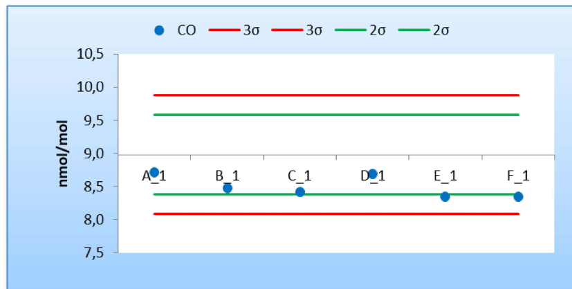
Figura 5 - Resultados y cumplimiento de los criterios de aceptación de sesgo de los laboratorios participantes para la concentración c4 de CO (8,98 \mu\text{mol/mol} )
