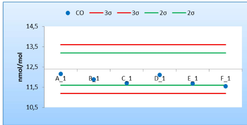
Figura 4 - Resultados y cumplimiento de los criterios de aceptación de sesgo de los laboratorios participantes para la concentración c3 de CO (12,39 \mu\text{mol/mol} )
