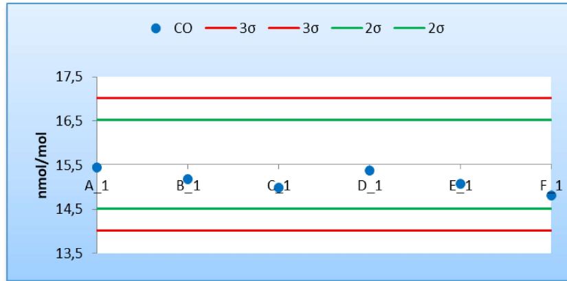
Figura 2 - Resultados y cumplimiento de los criterios de aceptación de sesgo de los laboratorios participantes para la concentración c1 de CO (15,52 µmol/mol)
