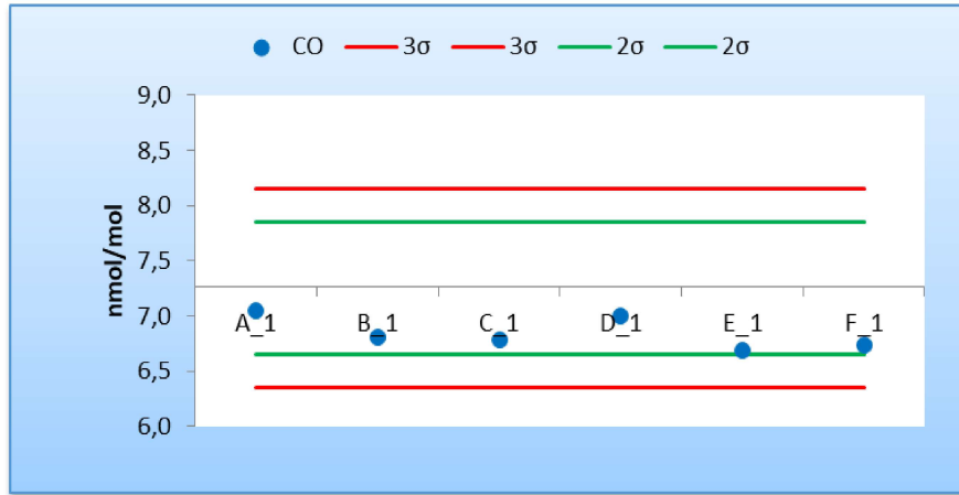
Figura 6 - Resultados y cumplimiento de los criterios de aceptación de sesgo de los laboratorios participantes para la concentración c5 de CO (7,26 \mu\text{mol/mol} )
