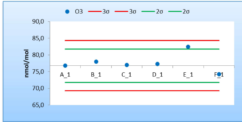
Figura 10 - Resultados y cumplimiento de los criterios de aceptación de sesgo de los laboratorios participantes para la concentración c4 de O 3 (76,81 nmol/mol)
