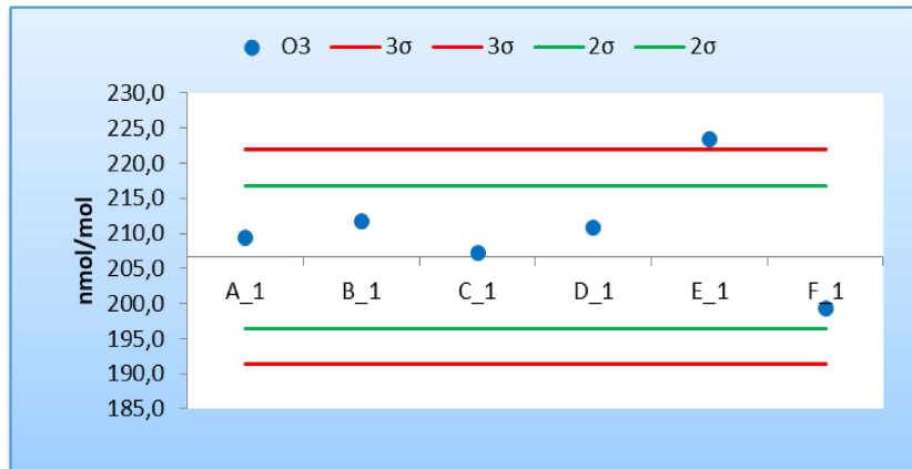
Figura 11 - Resultados y cumplimiento de los criterios de aceptación de sesgo de los laboratorios participantes para la concentración c5 de O 3 (206,59 nmol/mol)
