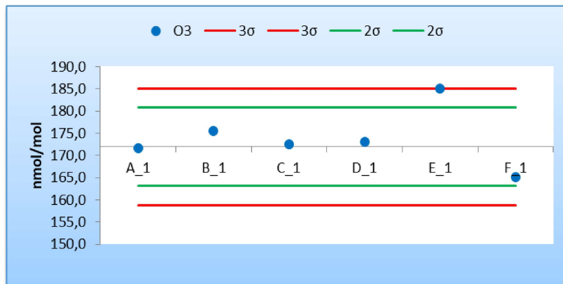
Figura 7 - Resultados y cumplimiento de los criterios de aceptación de sesgo de los laboratorios participantes para la concentración c1 de O 3 (171,92 nmol/mol)
