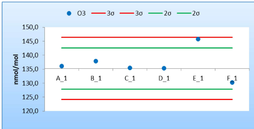
Figura 9 - Resultados y cumplimiento de los criterios de aceptación de sesgo de los laboratorios participantes para la concentración c3 de O 3 (135,22 nmol/mol)
