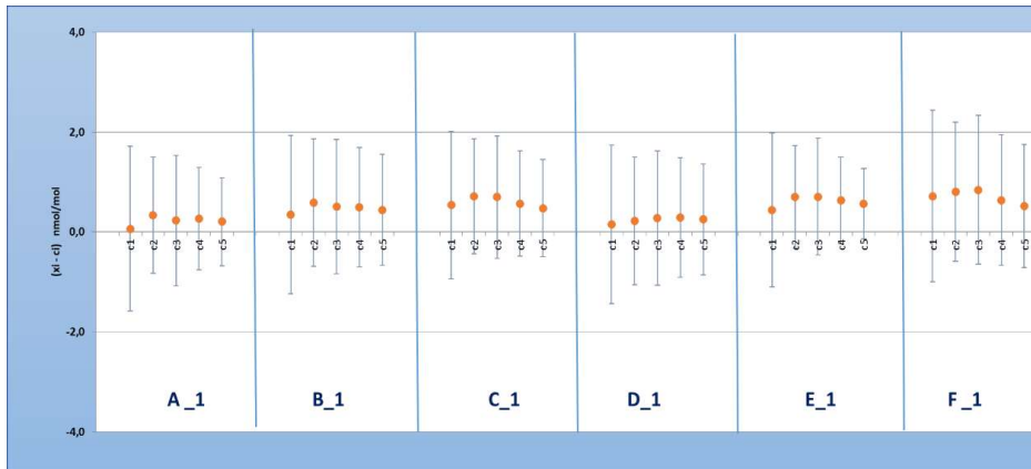
Figura 14.- Representación gráfica del sesgo de cada participante |x_i - c_i| con respecto al denominador de la ecuación del estadístico E_n para las concentraciones de CO
