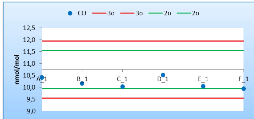
Figura 3 - Resultados y cumplimiento de los criterios de aceptación de sesgo de los laboratorios participantes para la concentración c2 de CO (10,75 µmol/mol)
