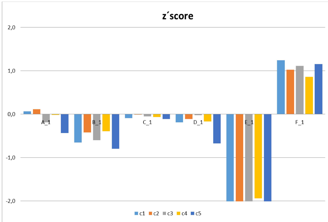
Figura 13 - Resultados de z´score para todos los participantes y todas las concentraciones de O 3 ensayadas
