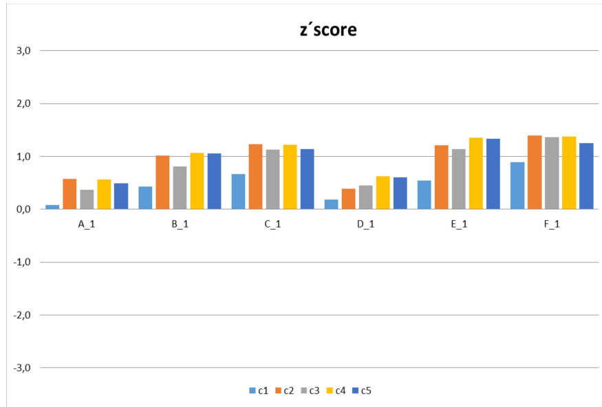
Figura 12 - Resultados de z´score para todos los participantes y todas las concentraciones de CO ensayadas
