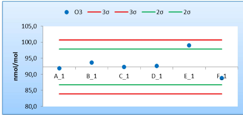
Figura 8 - Resultados y cumplimiento de los criterios de aceptación de sesgo de los laboratorios participantes para la concentración c2 de O 3 (92,29 nmol/mol)
