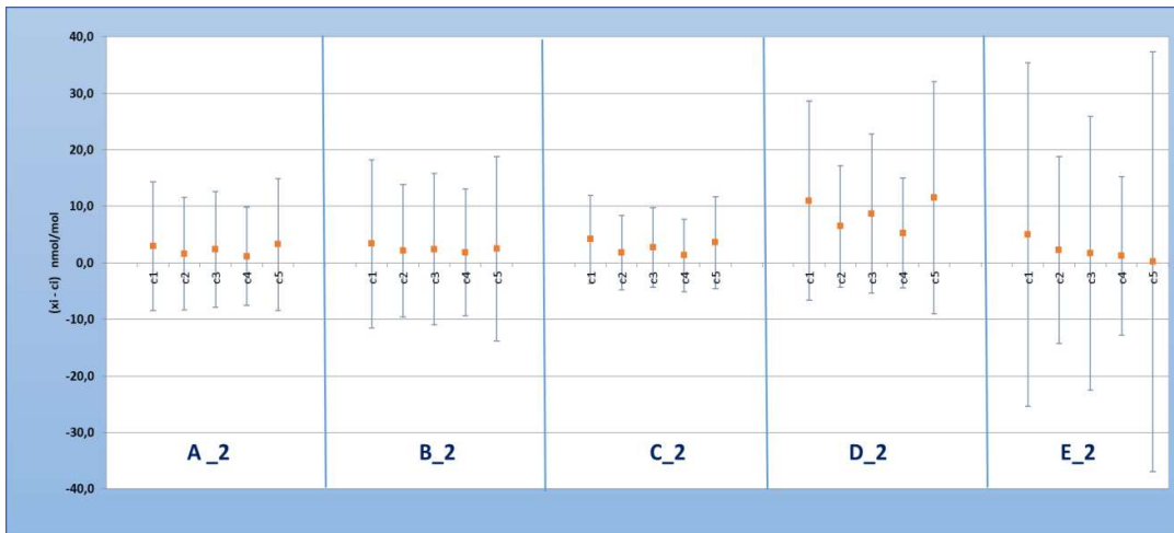
Figura 15.- Representación gráfica del sesgo de cada participante |x_i - c_i| con respecto al denominador de la ecuación del estadístico E_n para las concentraciones de O_3
