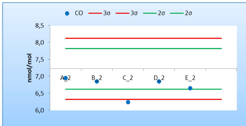
Figura 6 - Resultados y cumplimiento de los criterios de aceptación de sesgo de los laboratorios participantes para la concentración c5 de CO (7,23 \mu\text{mol/mol} )
