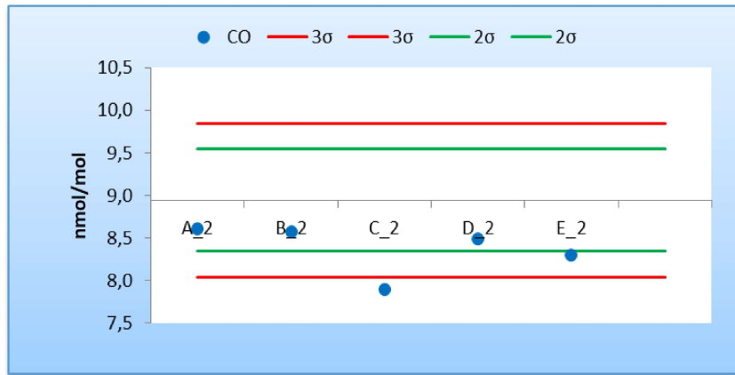
Figura 5 - Resultados y cumplimiento de los criterios de aceptación de sesgo de los laboratorios participantes para la concentración c4 de CO (8,94 \mu\text{mol/mol} )
