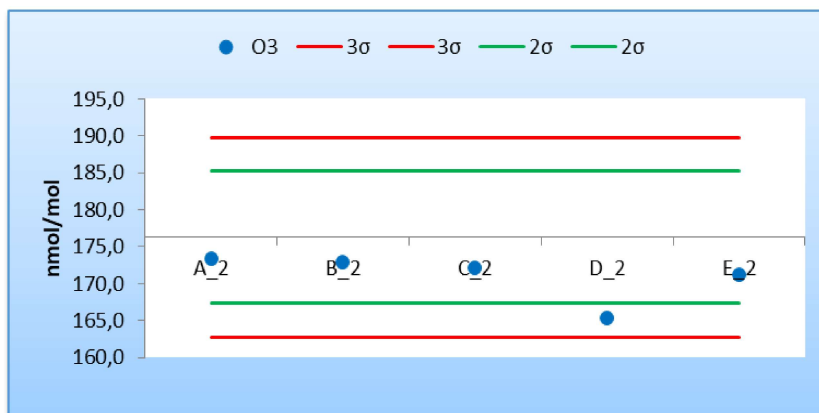
Figura 7 - Resultados y cumplimiento de los criterios de aceptación de sesgo de los laboratorios participantes para la concentración c1 de O 3 (176,29 nmol/mol)
