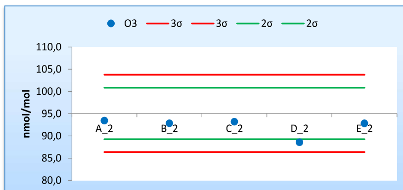
Figura 8 - Resultados y cumplimiento de los criterios de aceptación de sesgo de los laboratorios participantes para la concentración c2 de O 3 (95,06 nmol/mol)
