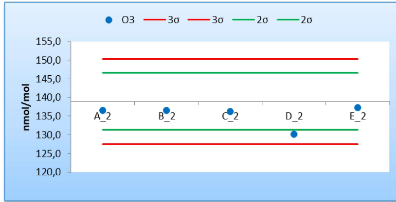
Figura 9 - Resultados y cumplimiento de los criterios de aceptación de sesgo de los laboratorios participantes para la concentración c3 de O 3 (138,97 nmol/mol)
