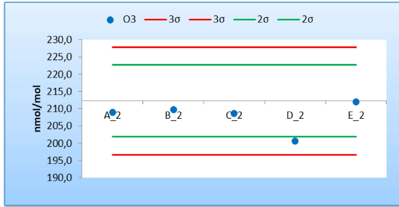
Figura 11 - Resultados y cumplimiento de los criterios de aceptación de sesgo de los laboratorios participantes para la concentración c5 de O 3 (212,26 nmol/mol)
