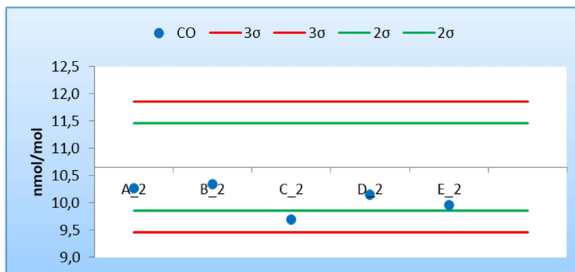
Figura 3 - Resultados y cumplimiento de los criterios de aceptación de sesgo de los laboratorios participantes para la concentración c2 de CO (10,65 \mu\text{mol/mol} )
