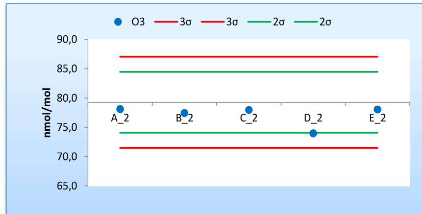
Figura 10 - Resultados y cumplimiento de los criterios de aceptación de sesgo de los laboratorios participantes para la concentración c4 de O 3 (79,28 nmol/mol)
