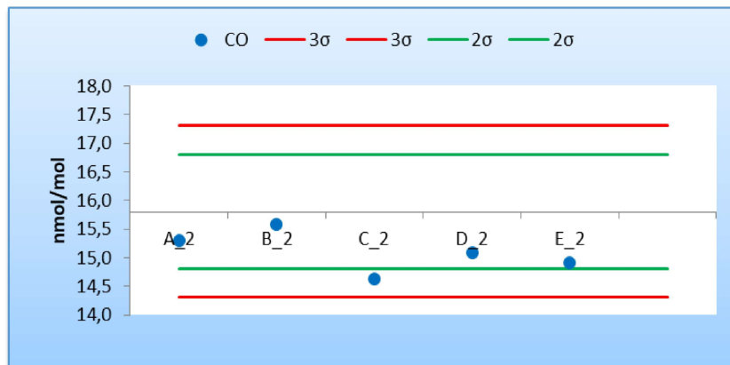
Figura 2 - Resultados y cumplimiento de los criterios de aceptación de sesgo de los laboratorios participantes para la concentración c1 de CO (15,80 μmol/mol)
