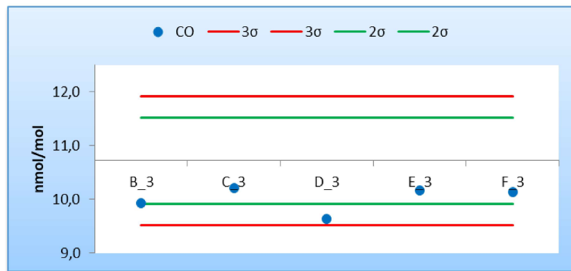
Figura 3 - Resultados y cumplimiento de los criterios de aceptación de sesgo de los laboratorios participantes para la concentración c2 de CO (10,72 μmol/mol)
