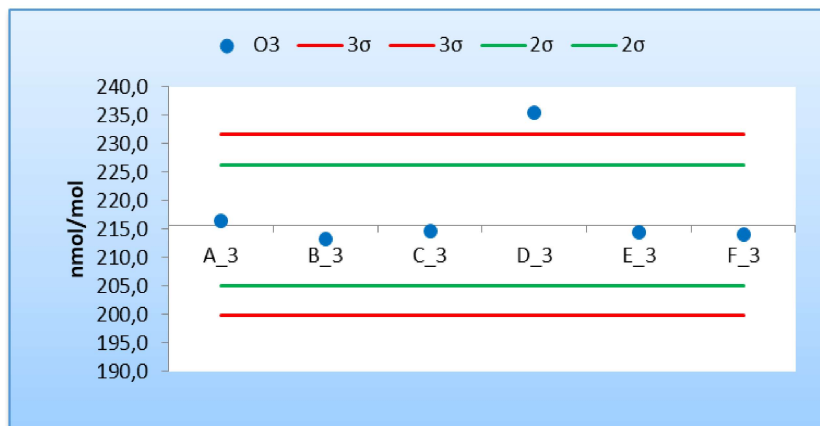
Figura 11 - Resultados y cumplimiento de los criterios de aceptación de sesgo de los laboratorios participantes para la concentración c5 de O 3 (215,75 nmol/mol)
