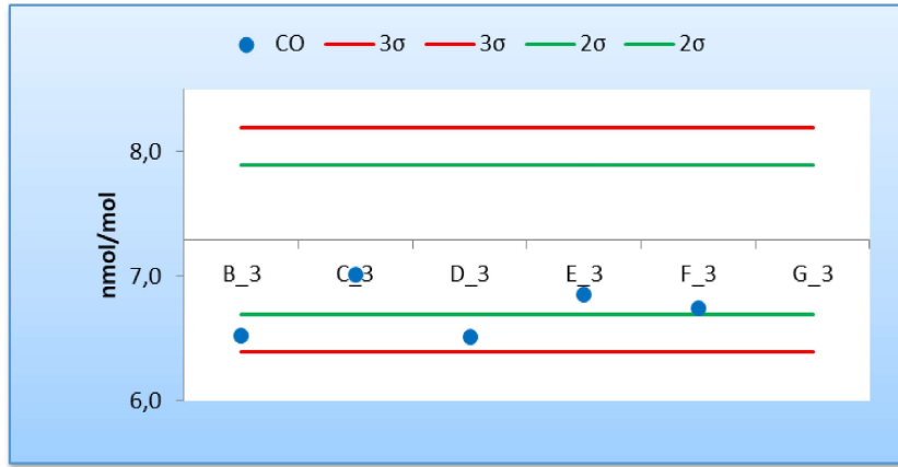
Figura 6 - Resultados y cumplimiento de los criterios de aceptación de sesgo de los laboratorios participantes para la concentración c5 de CO (7,29 \mu\text{mol/mol} )
