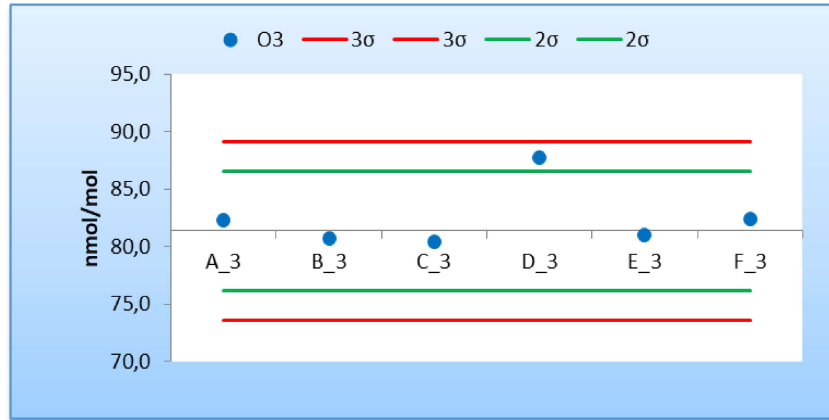
Figura 10 - Resultados y cumplimiento de los criterios de aceptación de sesgo de los laboratorios participantes para la concentración c4 de O 3 (81,37 nmol/mol)
