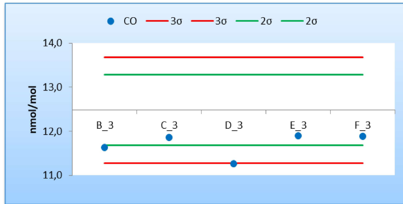
Figura 4 - Resultados y cumplimiento de los criterios de aceptación de sesgo de los laboratorios participantes para la concentración c3 de CO (12,48 \mu\text{mol/mol} )
