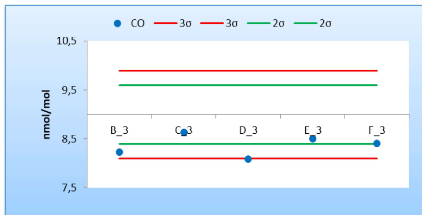
Figura 5 - Resultados y cumplimiento de los criterios de aceptación de sesgo de los laboratorios participantes para la concentración c4 de CO (9,00 \mu\text{mol/mol} )
