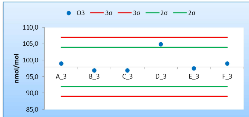
Figura 8 - Resultados y cumplimiento de los criterios de aceptación de sesgo de los laboratorios participantes para la concentración c2 de O 3 (97,95 nmol/mol)
