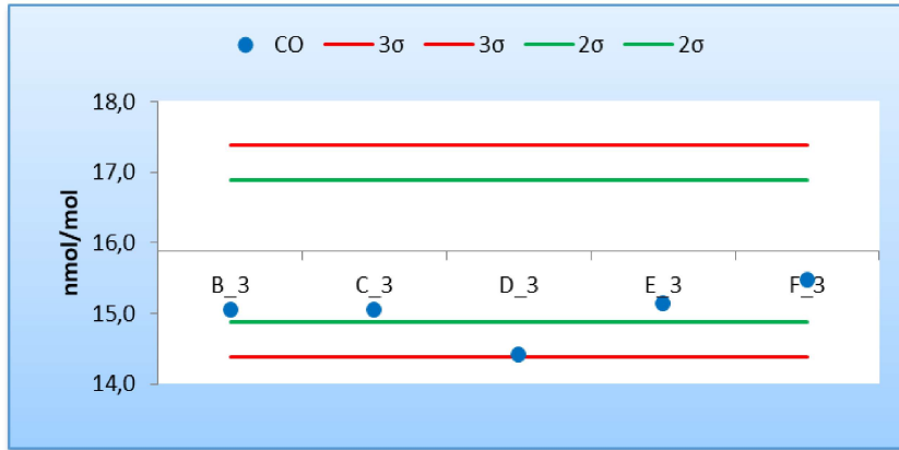
Figura 2 - Resultados y cumplimiento de los criterios de aceptación de sesgo de los laboratorios participantes para la concentración c1 de CO (15,88 μmol/mol)
