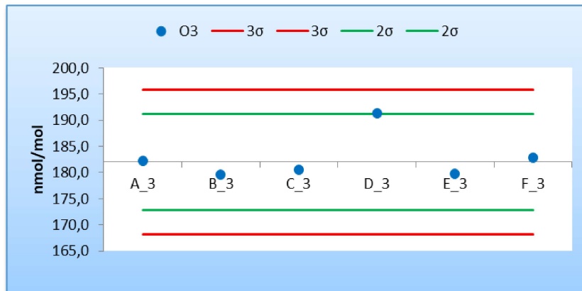
Figura 7 - Resultados y cumplimiento de los criterios de aceptación de sesgo de los laboratorios participantes para la concentración c1 de O 3 (182,03 nmol/mol)
