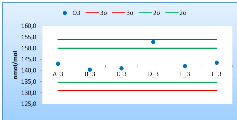
Figura 9 - Resultados y cumplimiento de los criterios de aceptación de sesgo de los laboratorios participantes para la concentración c3 de O 3 (142,39 nmol/mol)
